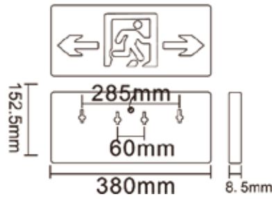
单面壁挂
