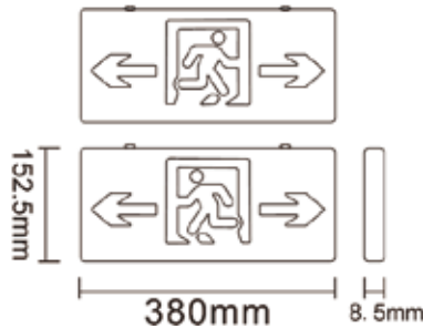
双面吊装
