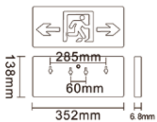
单面壁挂
